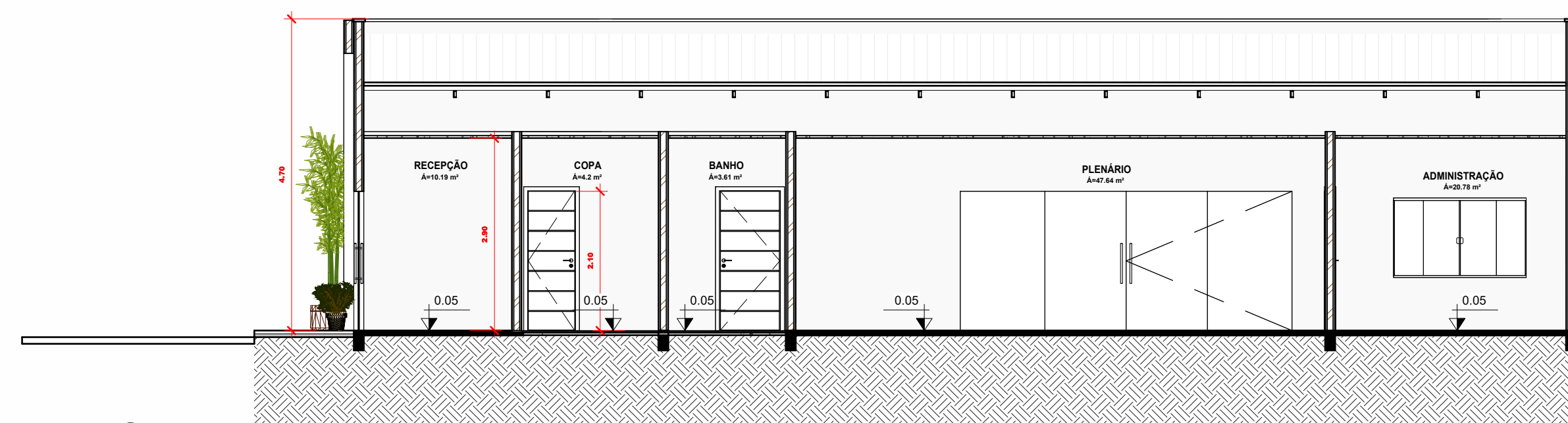
6 Corte AA 1 : 75
