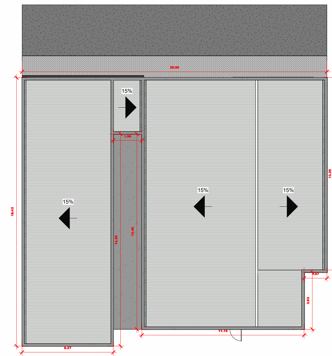
5 Planta da Cobertura 1 : 150
