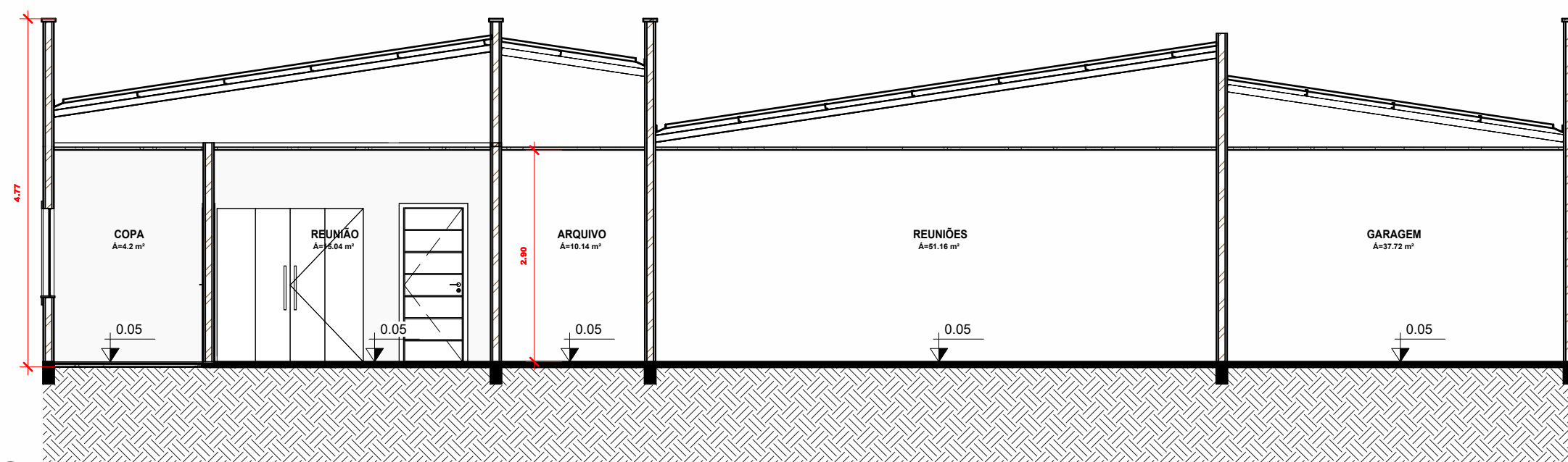
7 Corte BB 1 : 75
