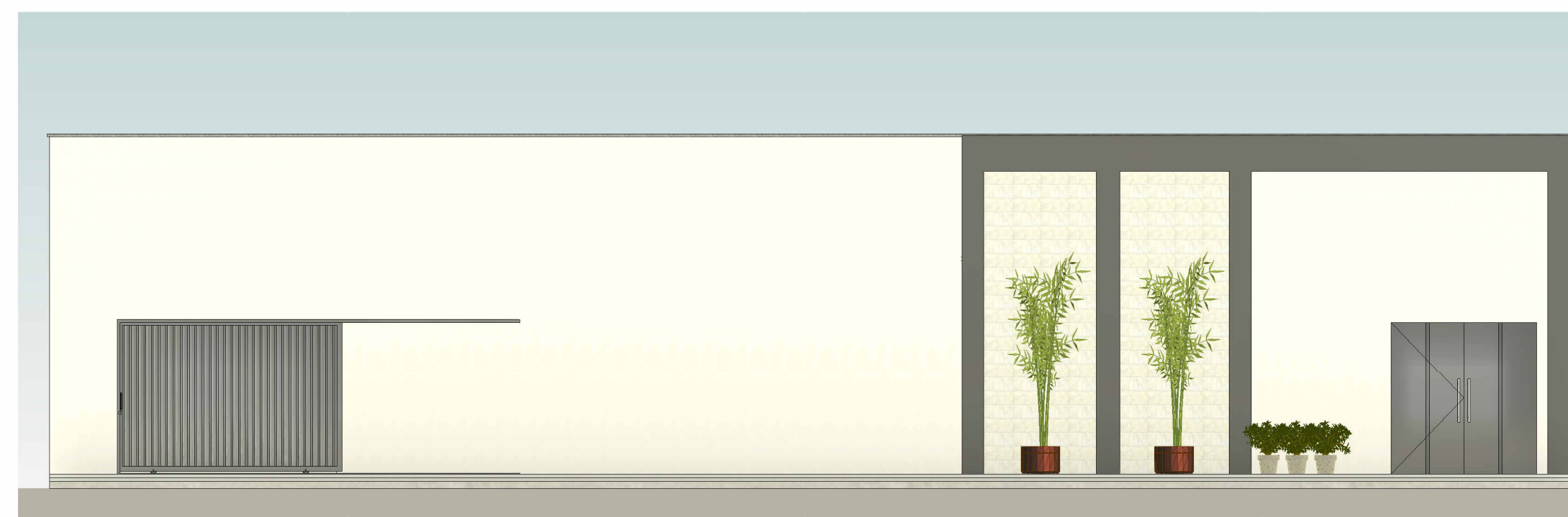
9 Elevação Frontal 1 : 75
