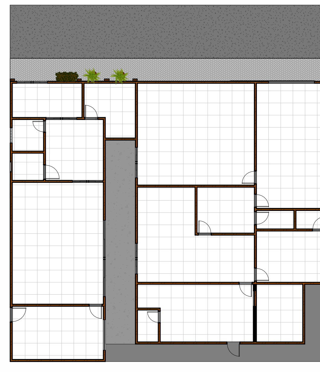
4 Planta Baixa - LAYOUT 1 : 150
