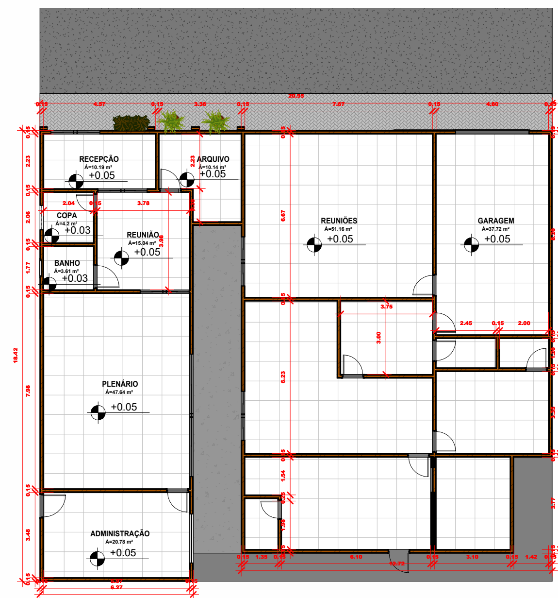
3 Planta Baixa - FUTURA 1 : 150
