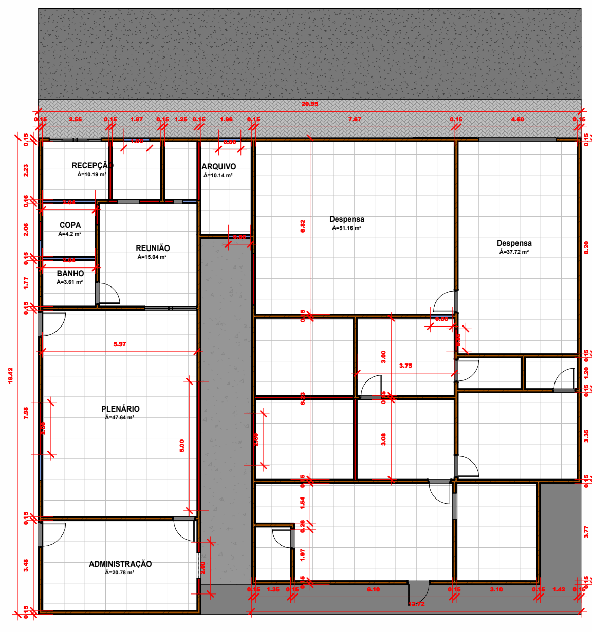
2 Planta Baixa - REFORMA 1 : 150
